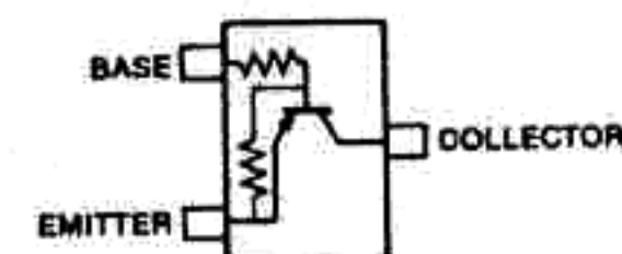
DTA144EU (Symbol: 16)
